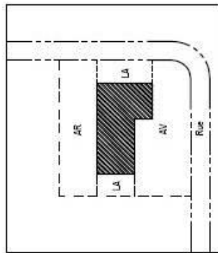
4. a) TERRAIN D'ANGLE
