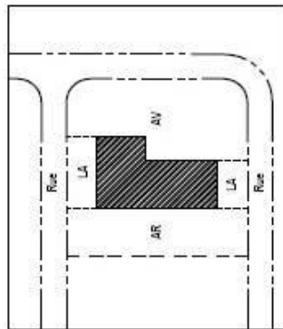
3. b) TERRAIN D'ANGLE TRANSVERSAL
