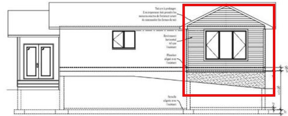
Élévation avant proposée
