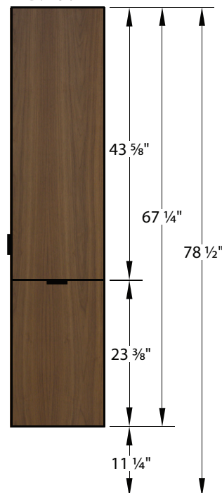
LINEN CAB. D: 16 1/4"
