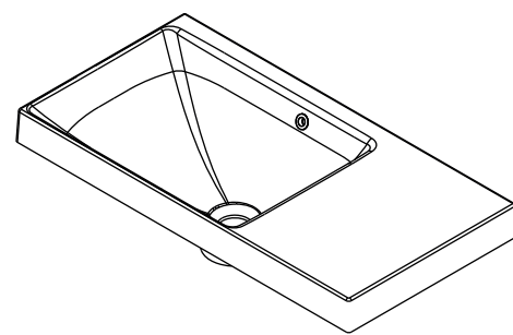
Lavabo MINI-12 DECENTRÉ GAUCHE 24 SINK SUR COMPTOIR / ABOVE-COUNTER MLOG0012-24 Dimensions extérieures : L 24 ¼" X I 12 ½" X H 6 ¼"
