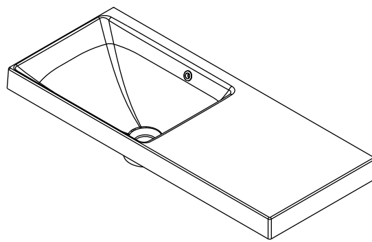
Lavabo MINI-12 DECENTRÉ GAUCHE 30 SINK SUR COMPTOIR / ABOVE-COUNTER MLOG0012-30 Dimensions extérieures : L 30 ¼" X I 12 ½" X H 6 ¼"
