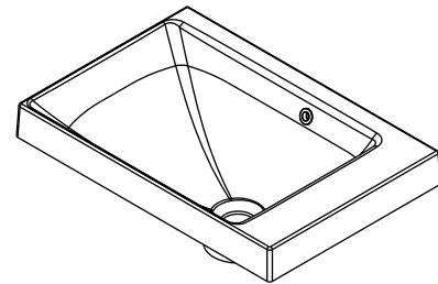
Lavabo MINI-12 DECENTRÉ GAUCHE 18 SINK SUR COMPTOIR / ABOVE-COUNTER MLOG0012-18 Dimensions extérieures : L 18 ¼" X I 12 ½" X H 6 ¼"
